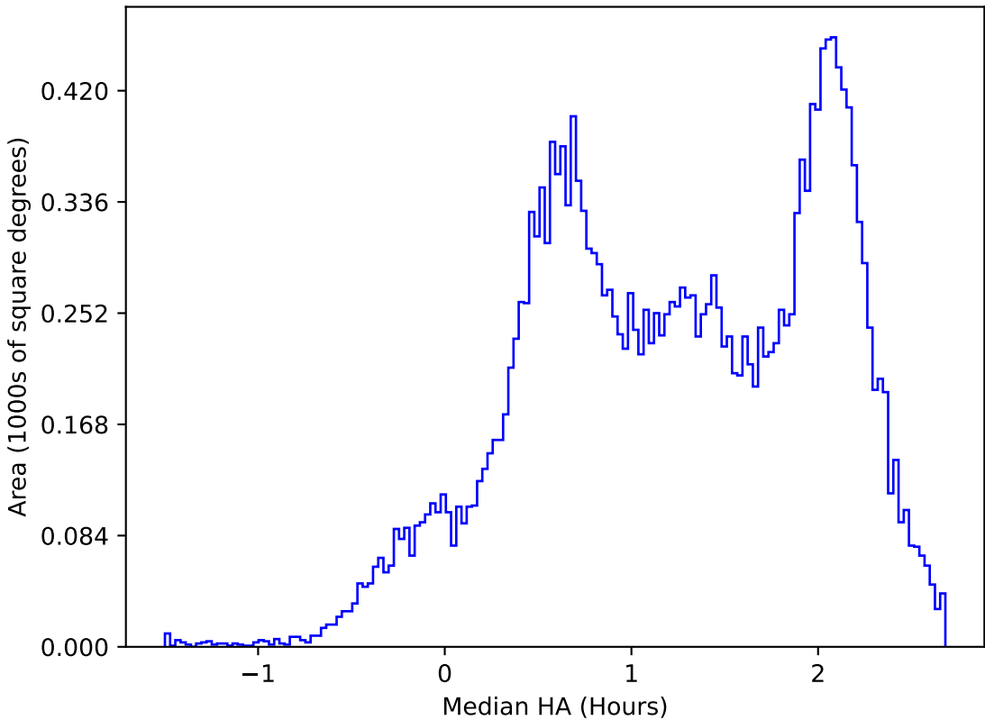
too_elab_r16_d2_ugrizy_v3.4_10yrs All sky y band: Median HA
