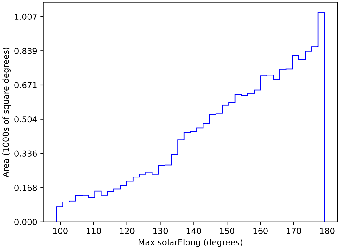
too_elab_r16_d2_ugrizy_v3.4_10yrs WFD y band: Max solarElong
