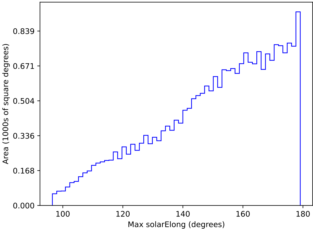
too_elab_r16_d2_ugrizy_v3.4_10yrs All sky y band: Max solarElong
