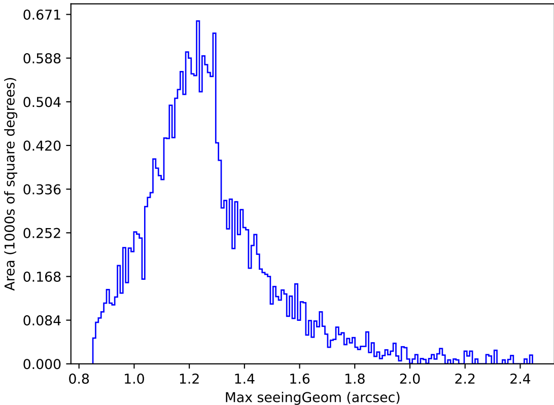
too_elab_r16_d2_ugrizy_v3.4_10yrs Yr 1 y band: Max seeingGeom
