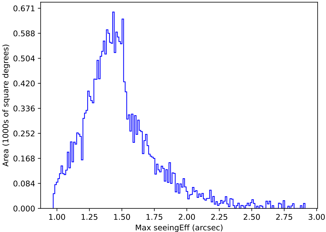
too_elab_r16_d2_ugrizy_v3.4_10yrs Yr 1 y band: Max seeingEff
