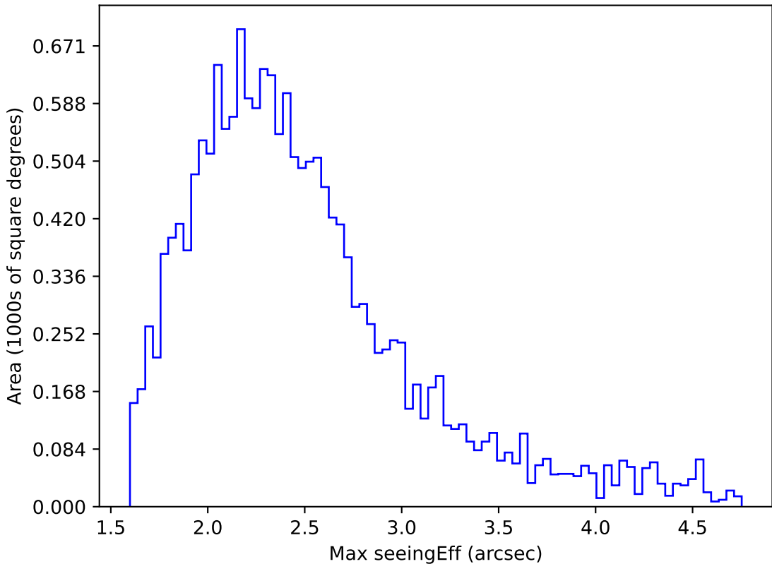
too_elab_r16_d2_ugrizy_v3.4_10yrs WFD y band: Max seeingEff
