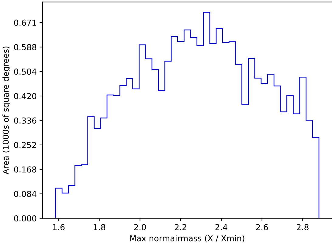
too_elab_r16_d2_ugrizy_v3.4_10yrs WFD z band: Max normairmass
