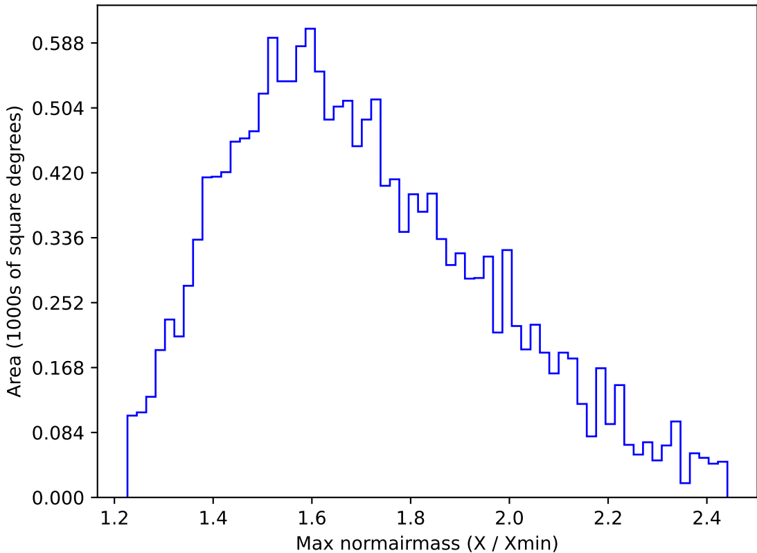
too_elab_r16_d2_ugrizy_v3.4_10yrs WFD u band: Max normairmass
