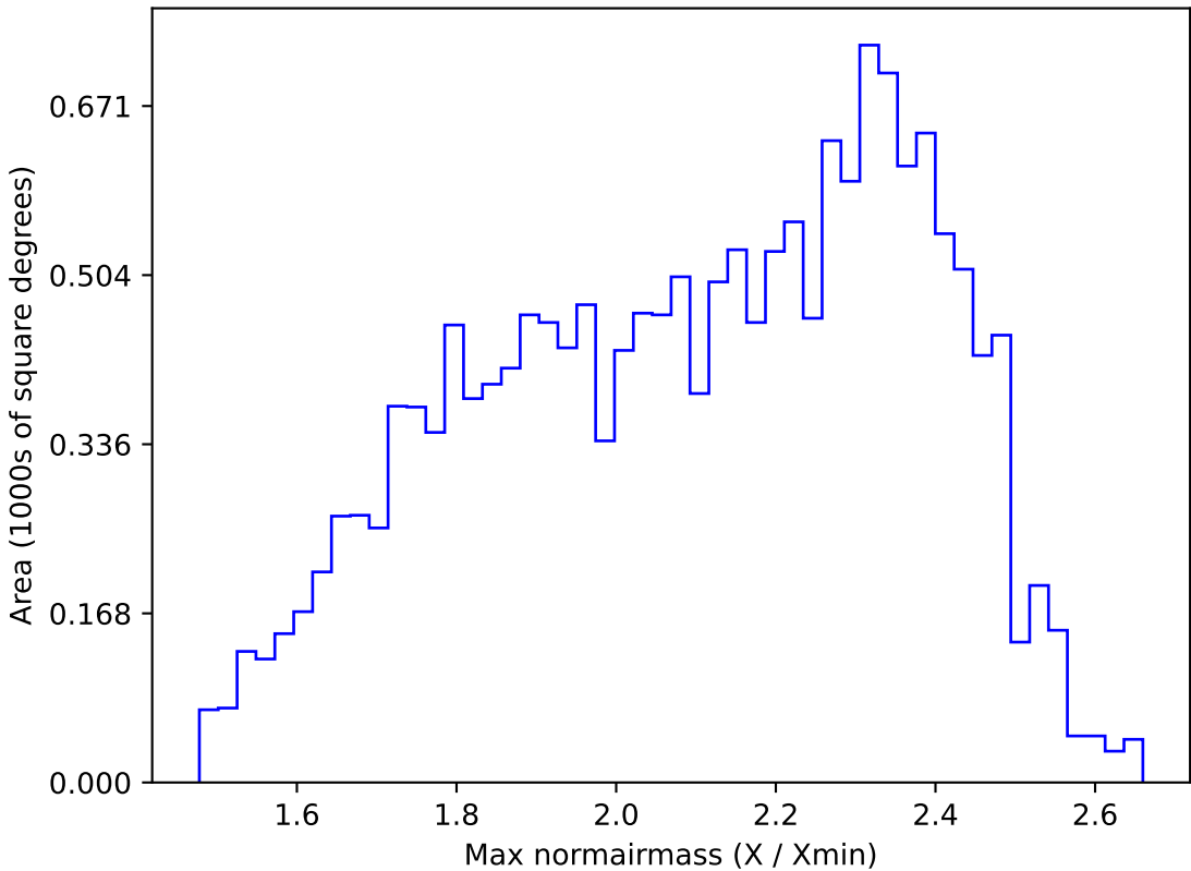
too_elab_r16_d2_ugrizy_v3.4_10yrs WFD r band: Max normairmass
