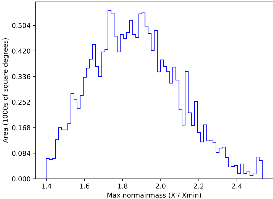
too_elab_r16_d2_ugrizy_v3.4_10yrs WFD g band: Max normairmass
