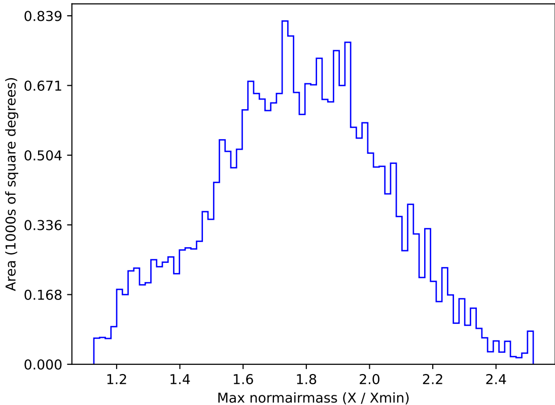
too_elab_r16_d2_ugrizy_v3.4_10yrs All sky g band: Max normairmass
