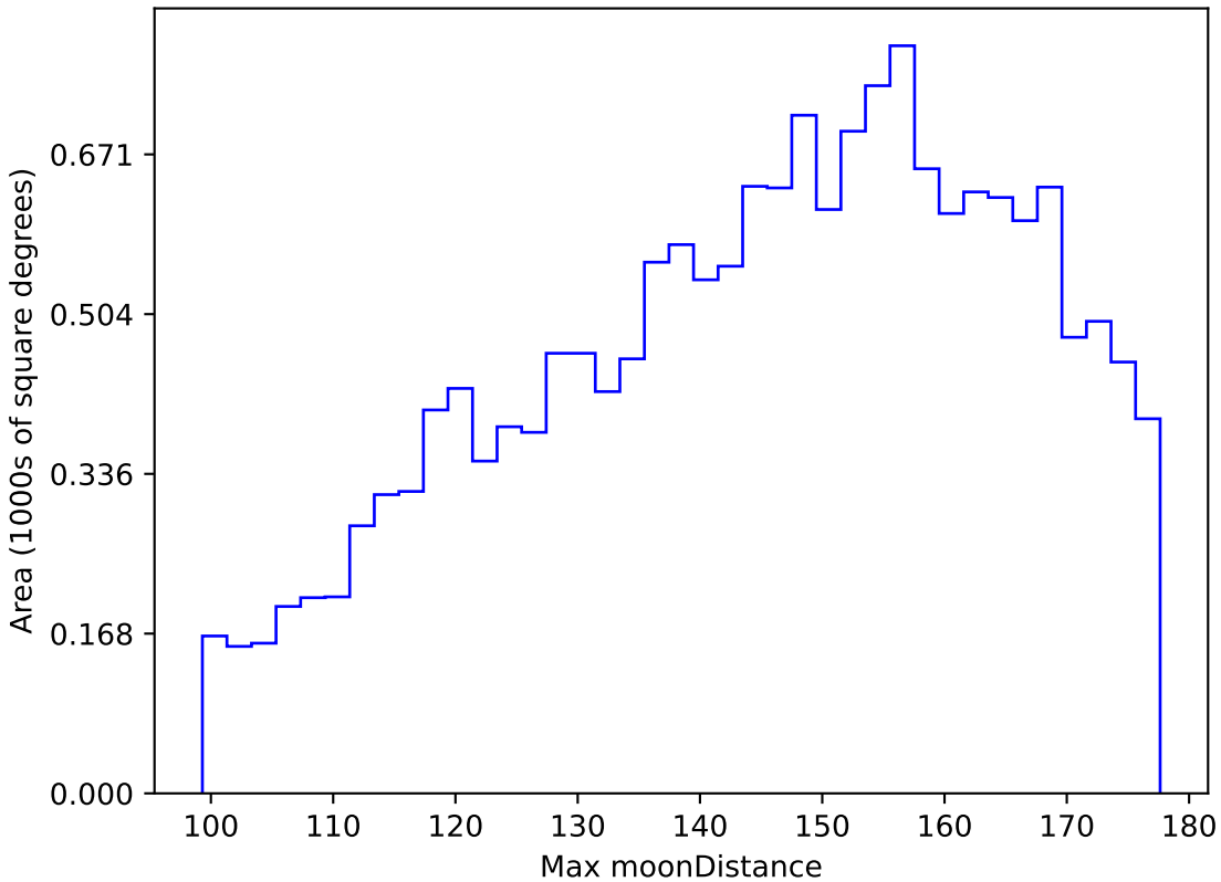
too_elab_r16_d2_ugrizy_v3.4_10yrs WFD y band: Max moonDistance
