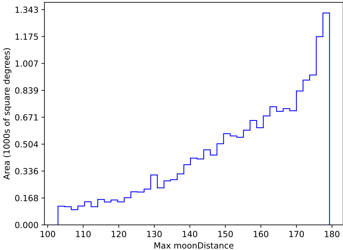
too_elab_r16_d2_ugrizy_v3.4_10yrs WFD i band: Max moonDistance
