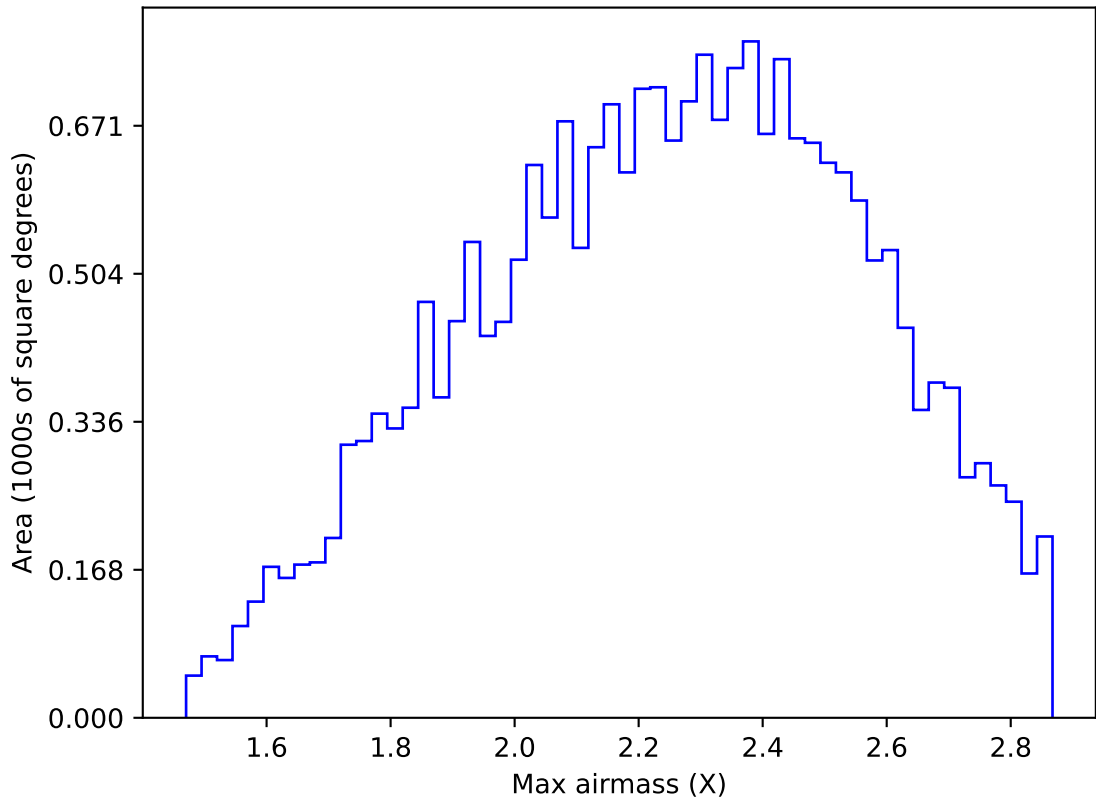
too_elab_r16_d2_ugrizy_v3.4_10yrs All sky y band: Max airmass
