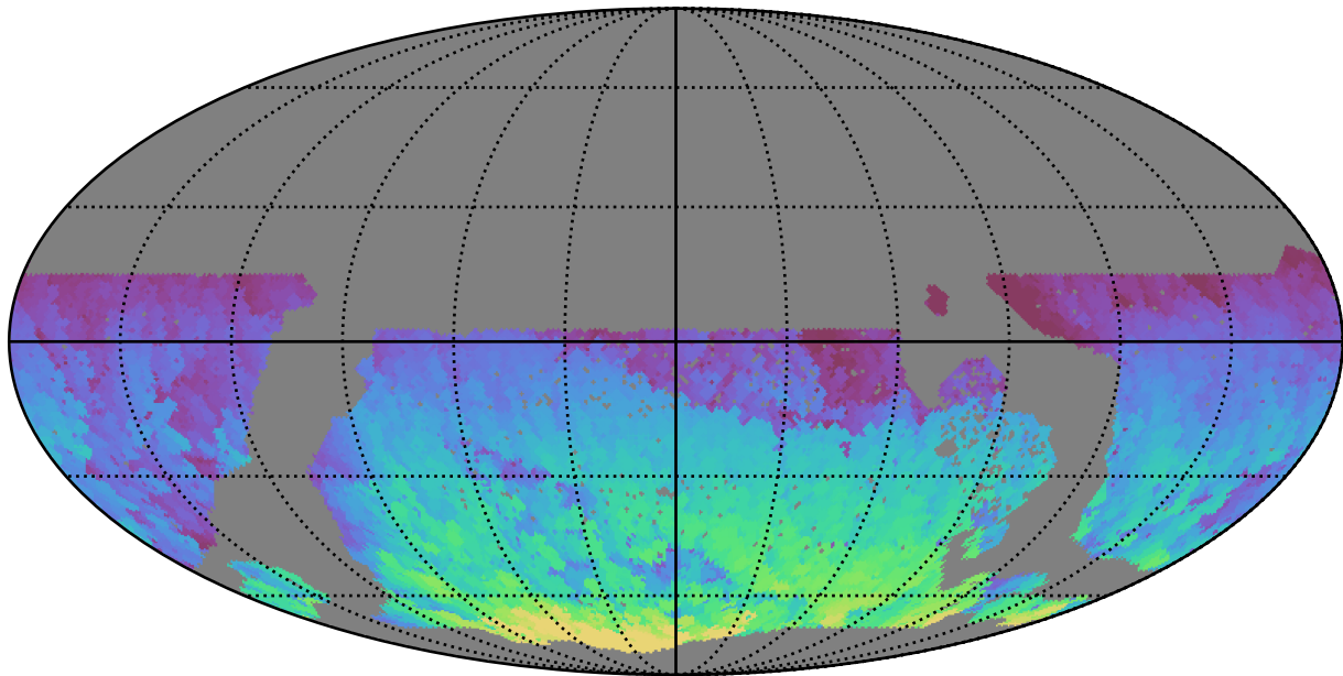
too_elab_r16_d2_ugrizy_v3.4_10yrs WFD z band: Max HA
