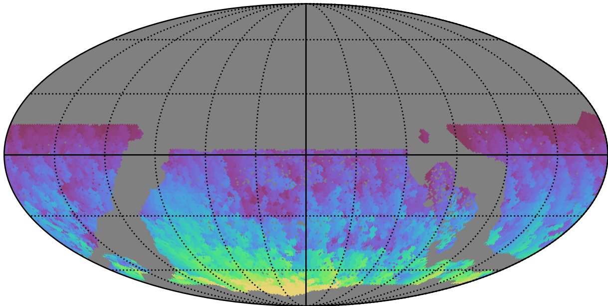
too_elab_r16_d2_ugrizy_v3.4_10yrs WFD y band: Max HA
