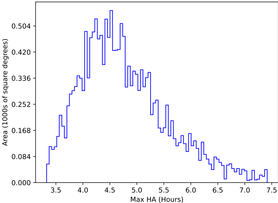
too_elab_r16_d2_ugrizy_v3.4_10yrs WFD y band: Max HA
