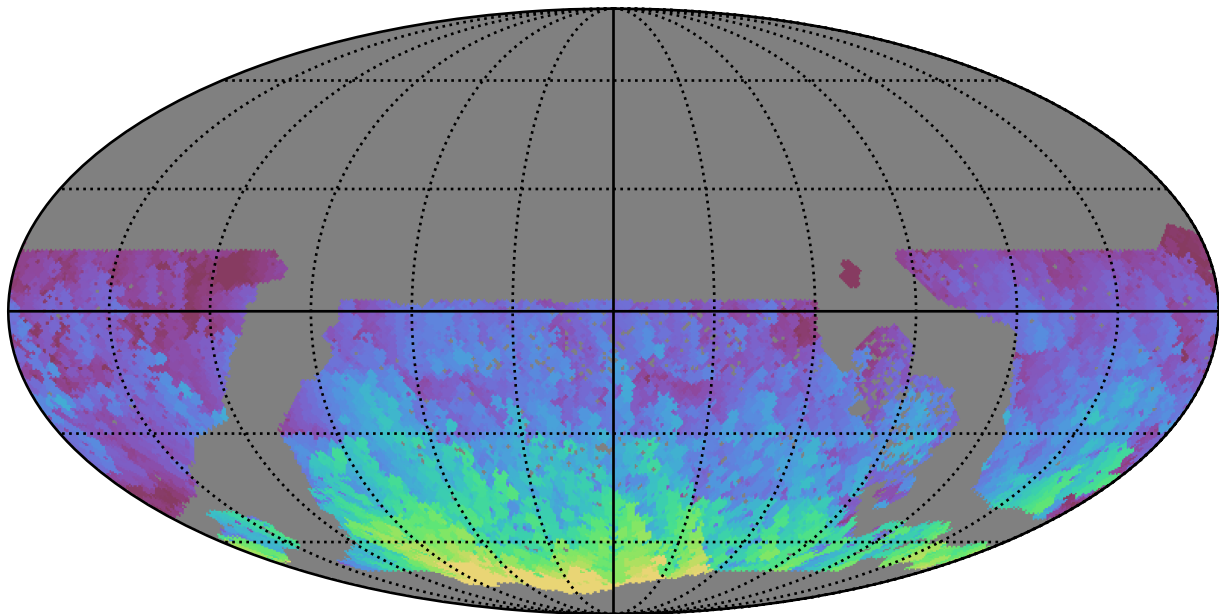
too_elab_r16_d2_ugrizy_v3.4_10yrs WFD r band: Max HA
