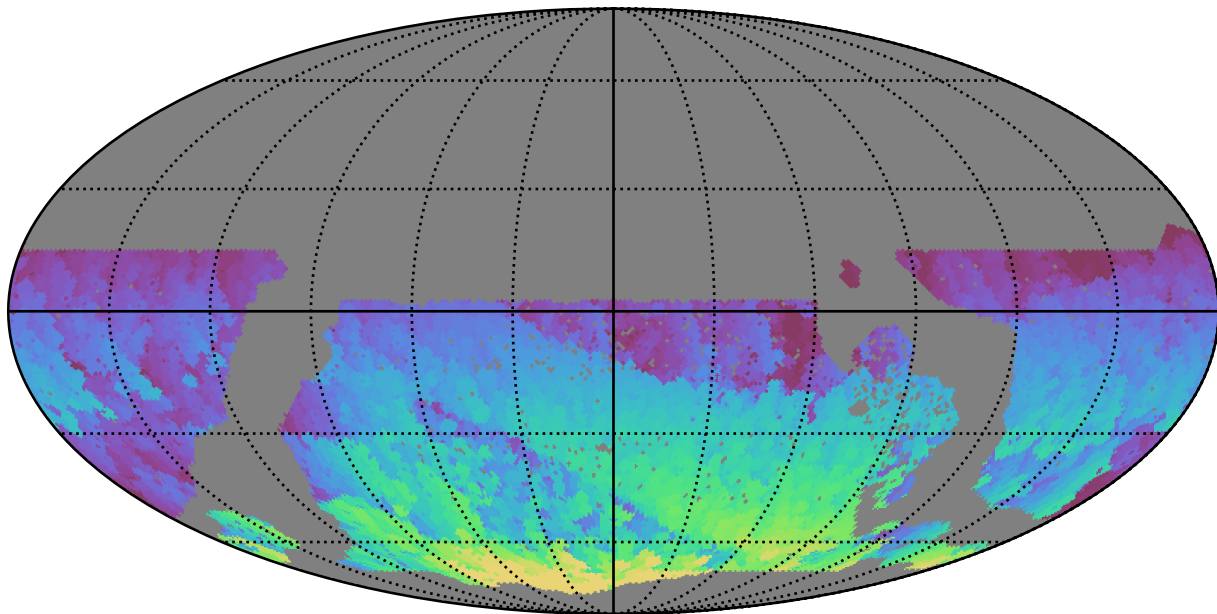
too_elab_r16_d2_ugrizy_v3.4_10yrs WFD i band: Max HA
