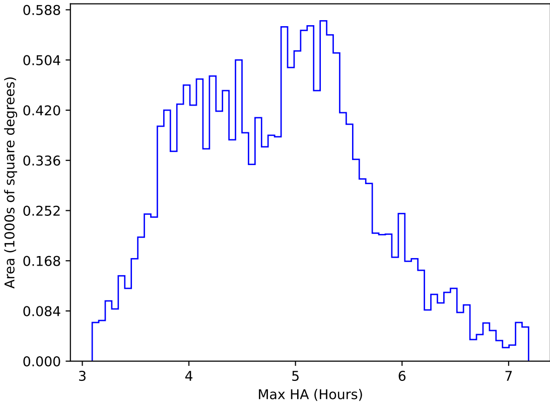
too_elab_r16_d2_ugrizy_v3.4_10yrs WFD i band: Max HA
