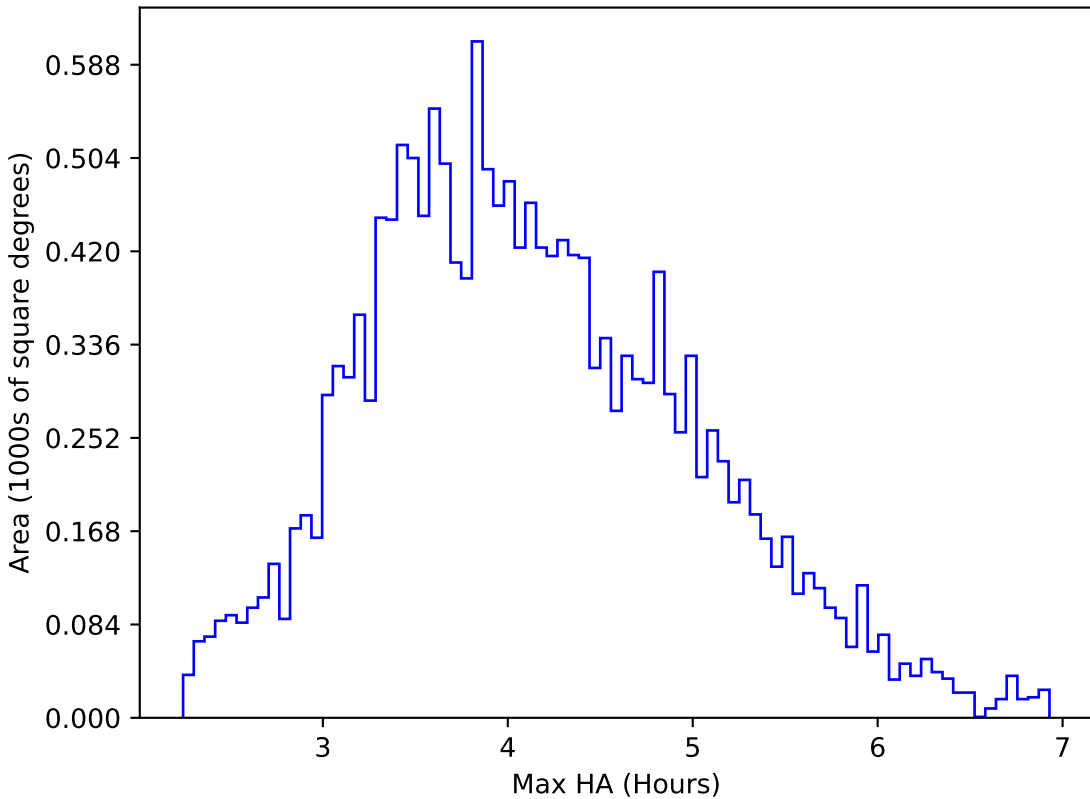
too_elab_r16_d2_ugrizy_v3.4_10yrs WFD g band: Max HA
