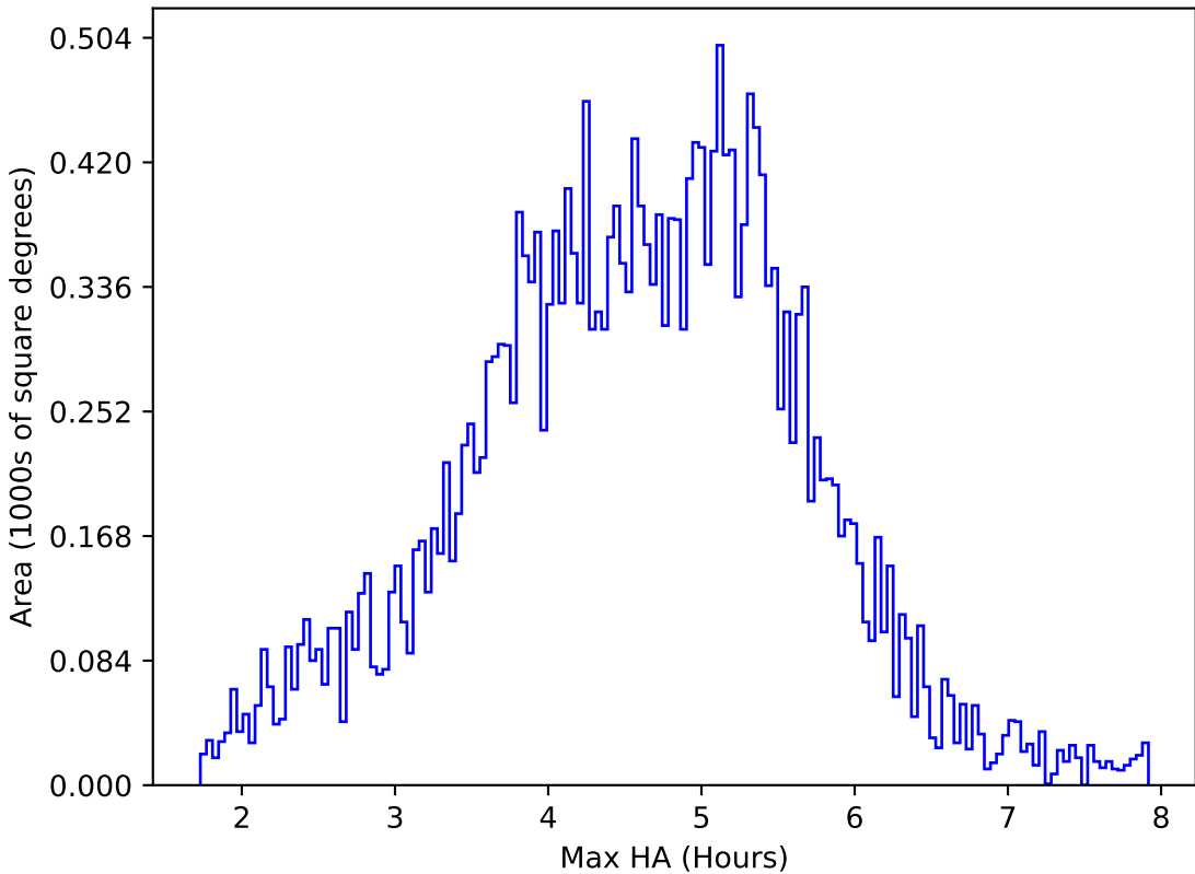
too_elab_r16_d2_ugrizy_v3.4_10yrs All sky z band: Max HA
