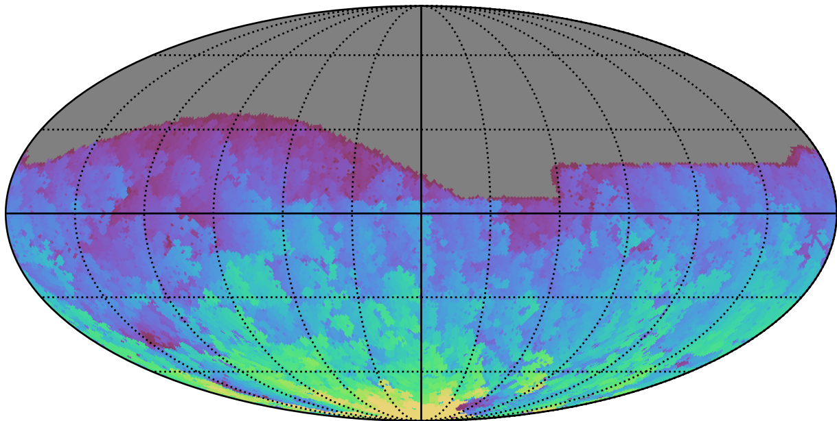
too_elab_r16_d2_ugrizy_v3.4_10yrs All sky g band: Max HA
