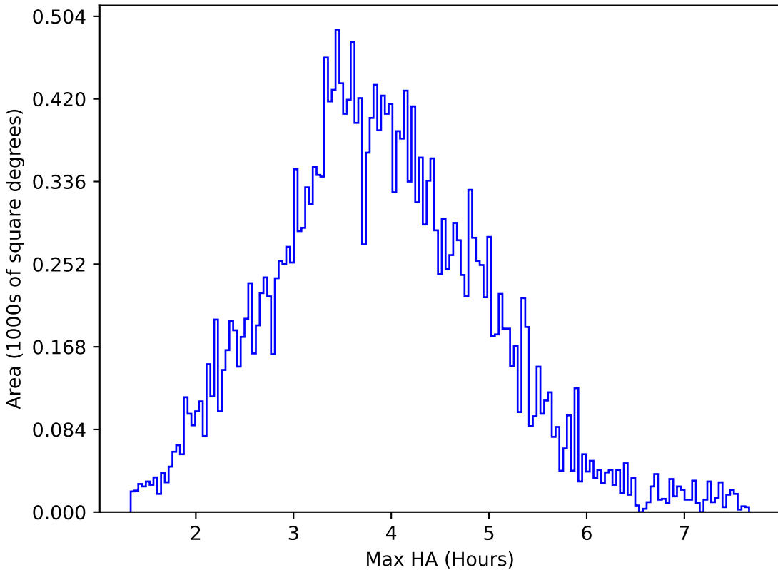
too_elab_r16_d2_ugrizy_v3.4_10yrs All sky g band: Max HA
