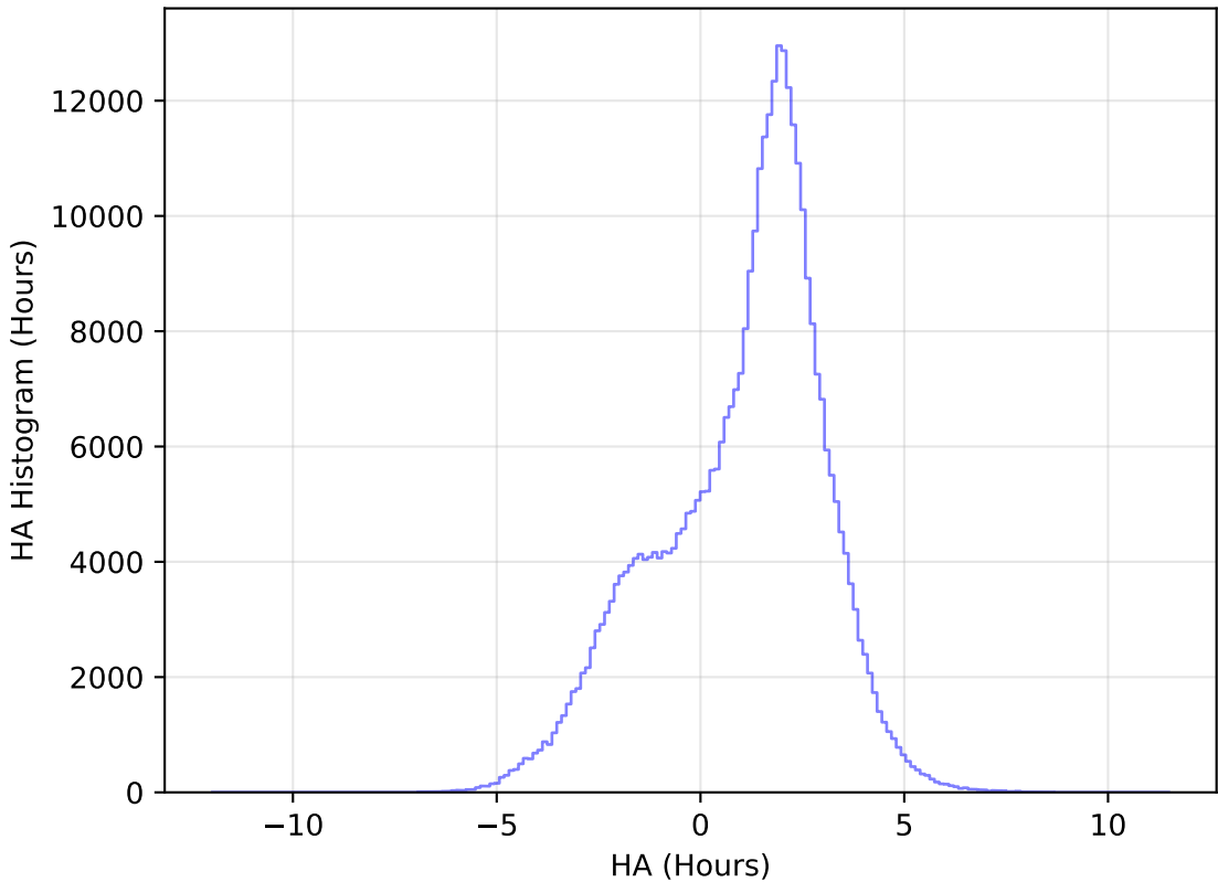
too_elab_r16_d2_ugrizy_v3.4_10yrs WFD y band: HA Histogram
