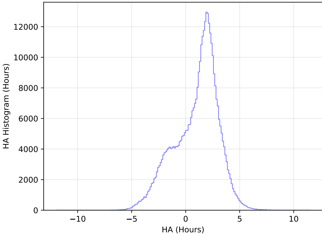
too_elab_r16_d2_ugrizy_v3.4_10yrs All sky y band: HA Histogram
