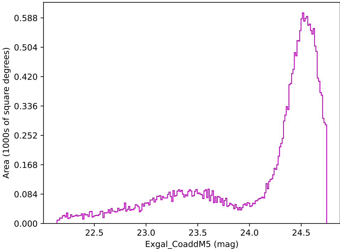
too_elab_r16_d2_ugrizy_v3.4_10yrs Yr 1 z band: Exgal_CoaddM5
