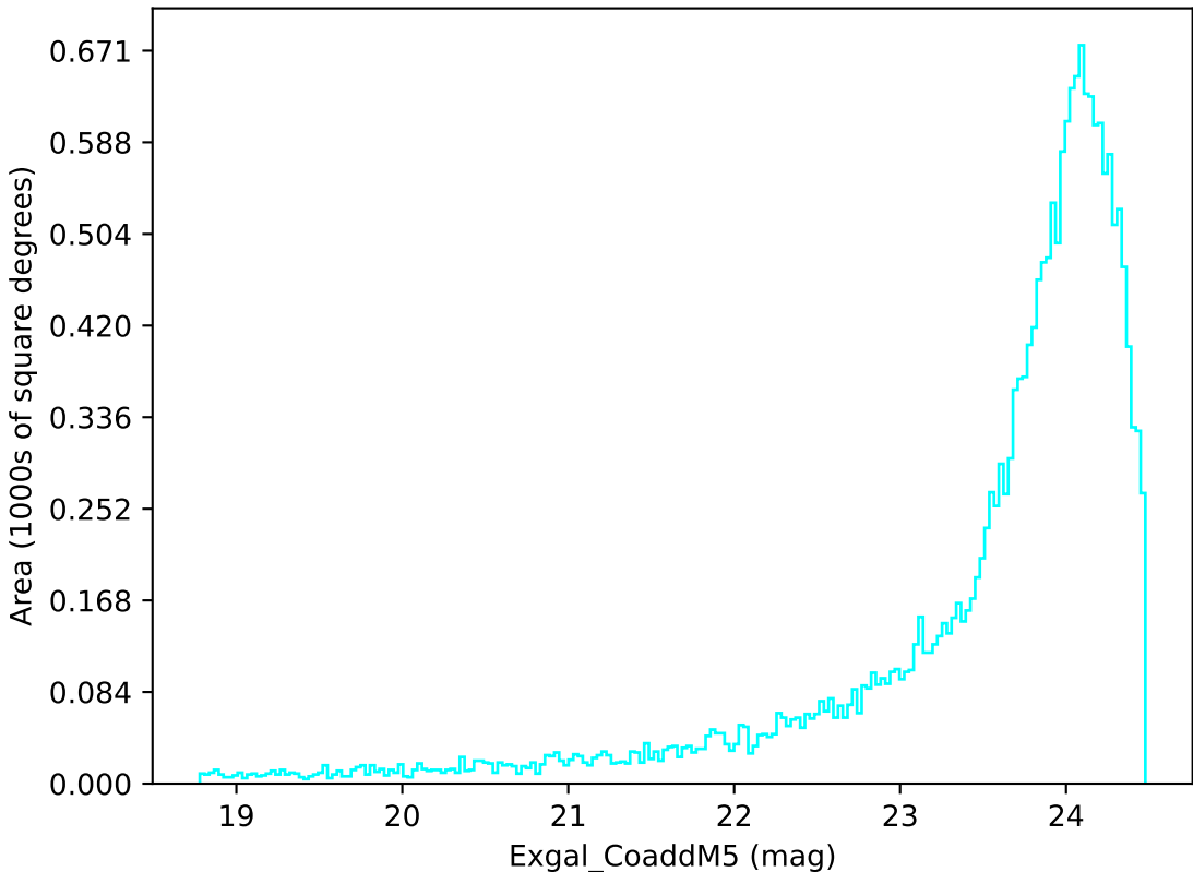
too_elab_r16_d2_ugrizy_v3.4_10yrs Yr 1 u band: Exgal_CoaddM5
