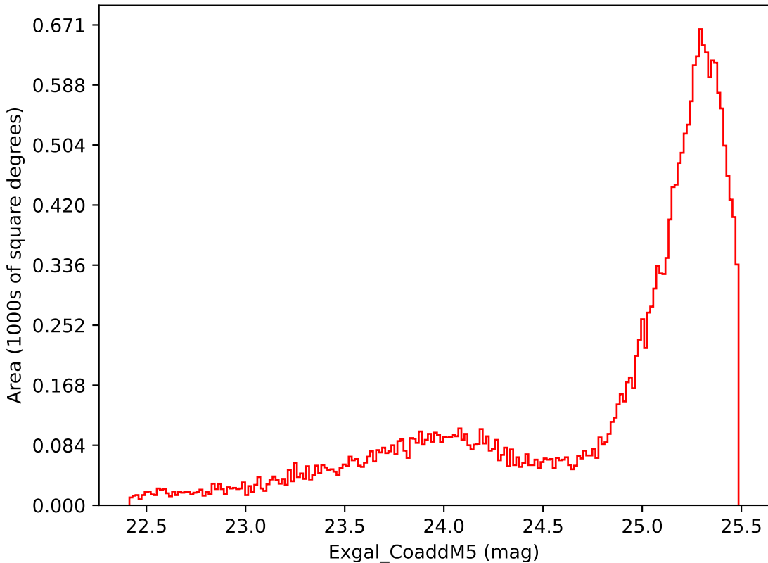
too_elab_r16_d2_ugrizy_v3.4_10yrs Yr 1 i band: Exgal_CoaddM5
