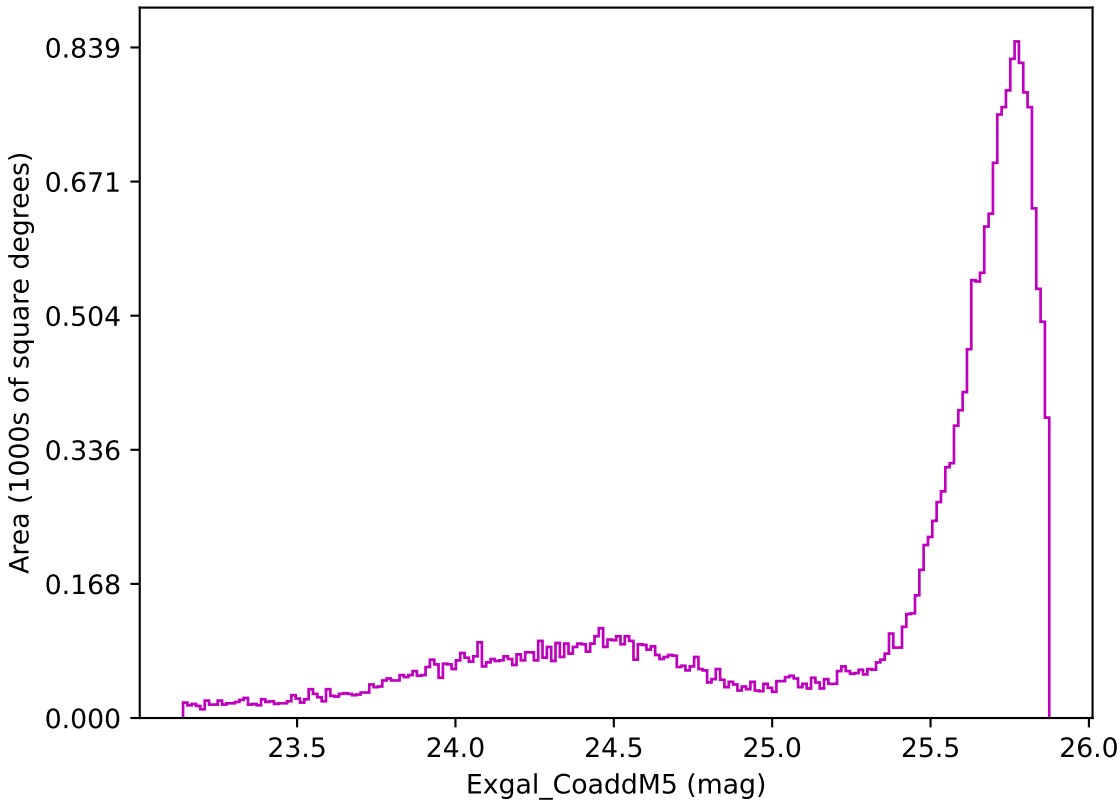
too_elab_r16_d2_ugrizy_v3.4_10yrs All sky z band: Exgal_CoaddM5
