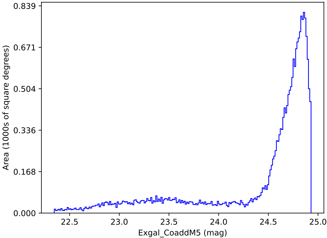
too_elab_r16_d2_ugrizy_v3.4_10yrs All sky y band: Exgal_CoaddM5
