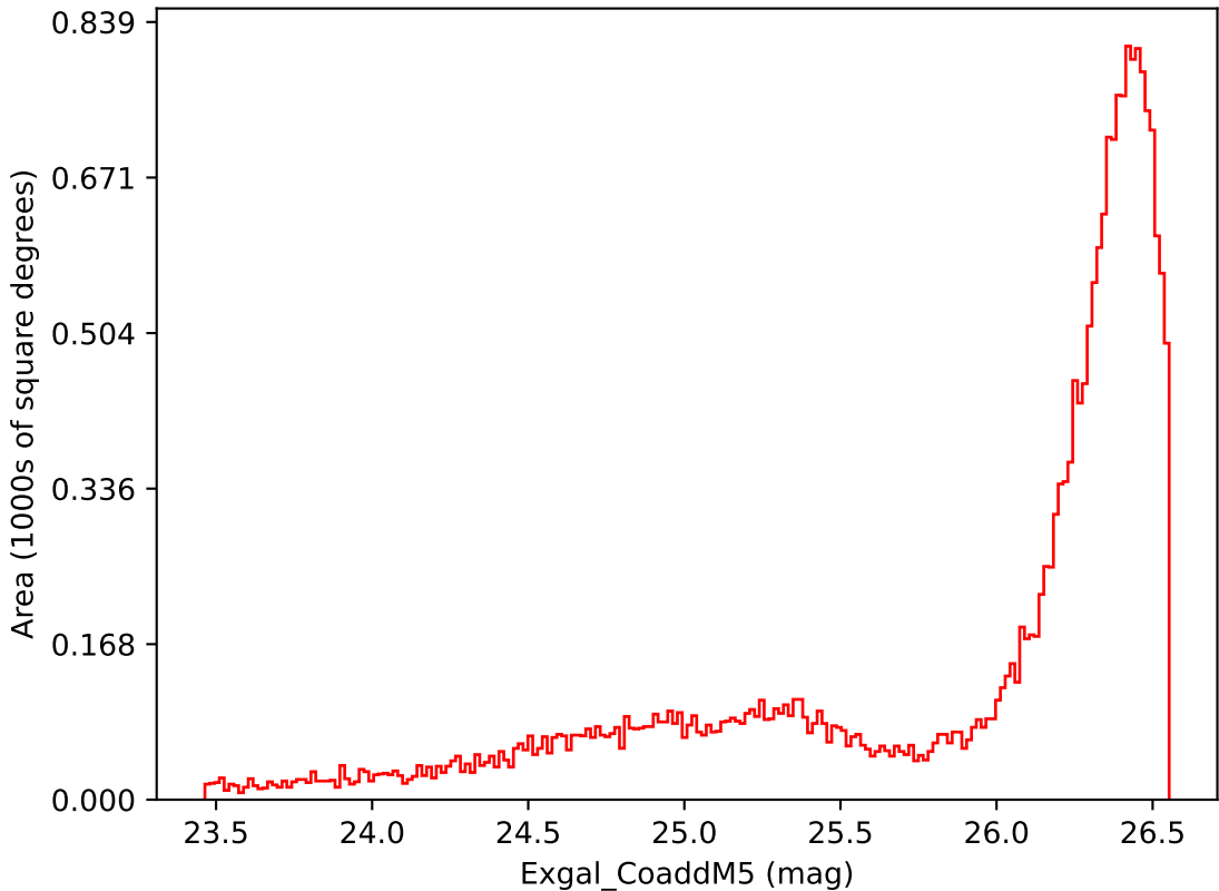
too_elab_r16_d2_ugrizy_v3.4_10yrs All sky i band: Exgal_CoaddM5
