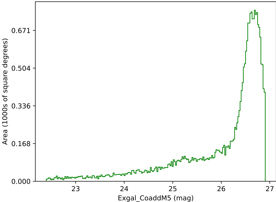
too_elab_r16_d2_ugrizy_v3.4_10yrs All sky g band: Exgal_CoaddM5
