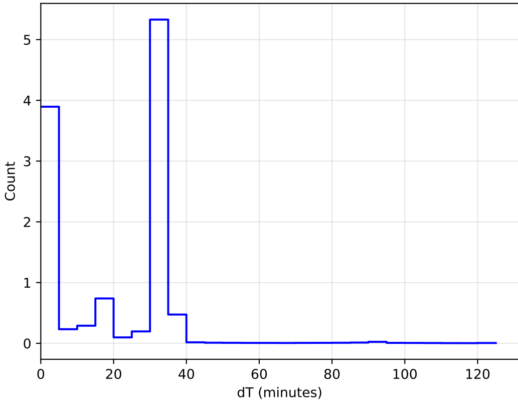
too_elab_r16_d2_ugrizy_v3.4_10yrs WFD: DeltaT Histogram 1e6
