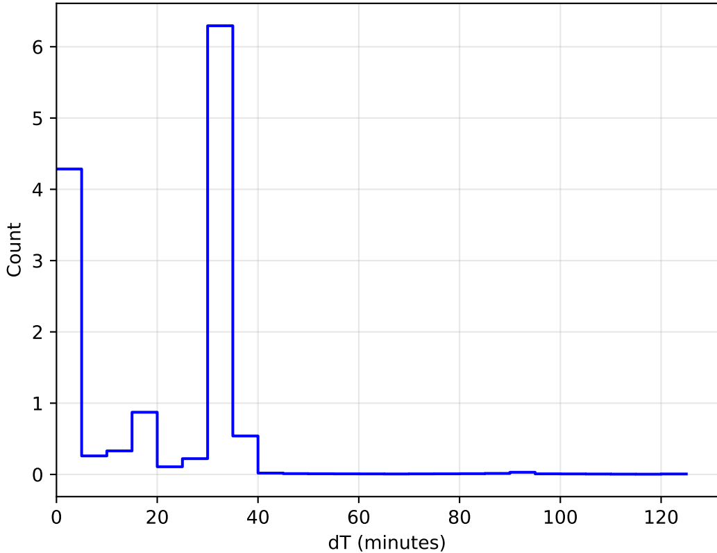
too_elab_r16_d2_ugrizy_v3.4_10yrs All sky: DeltaT Histogram 1e6
