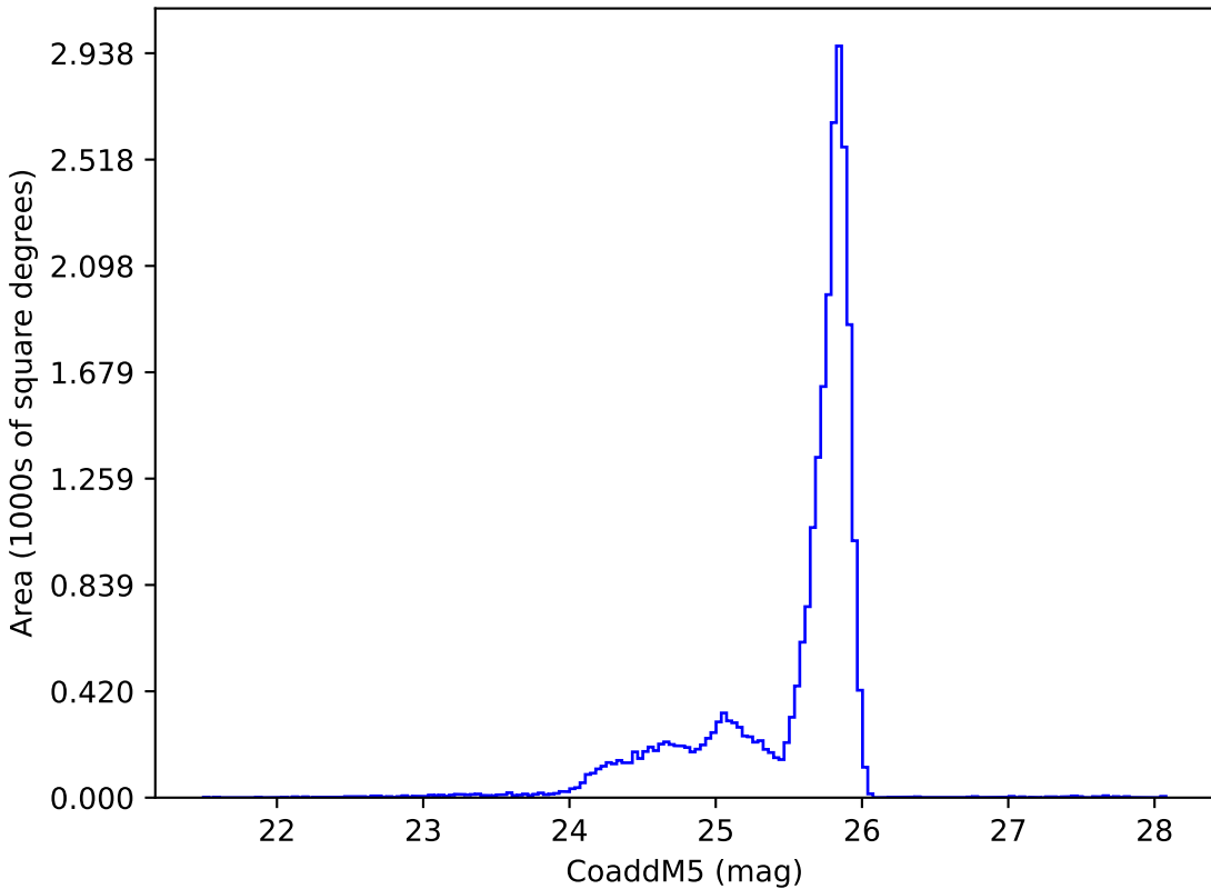
too_elab_r16_d2_ugrizy_v3.4_10yrs z: CoaddM5
