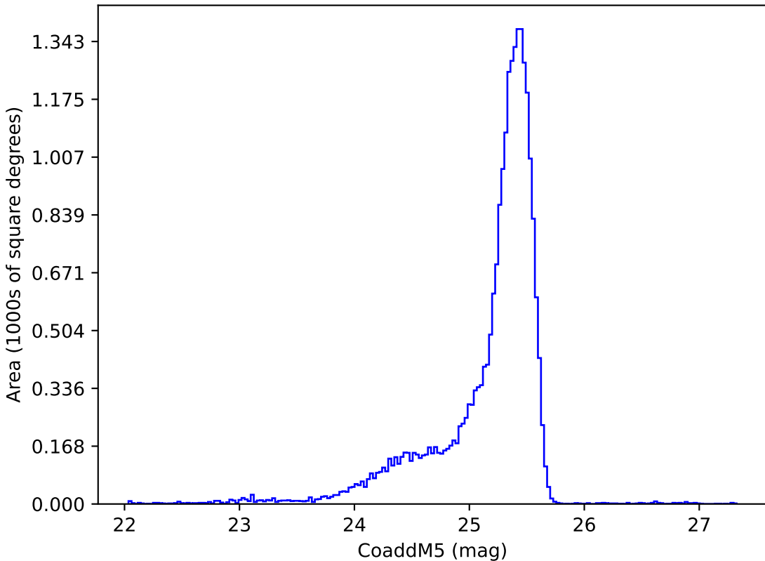
too_elab_r16_d2_ugrizy_v3.4_10yrs u: CoaddM5
