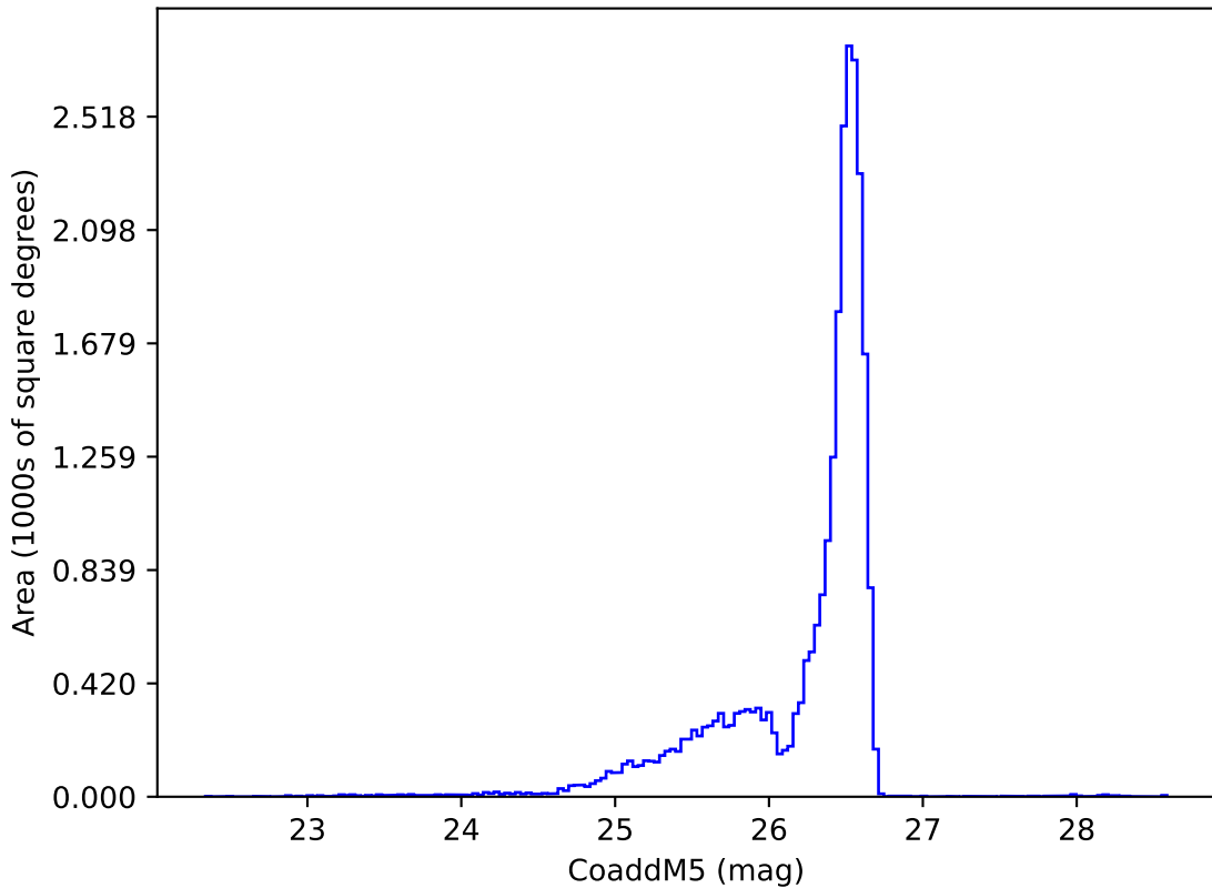
too_elab_r16_d2_ugrizy_v3.4_10yrs i: CoaddM5
