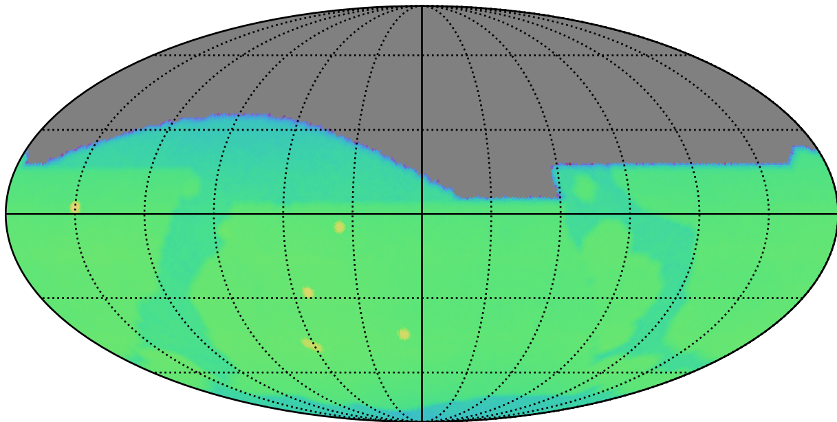
too_elab_r16_d2_ugrizy_v3.4_10yrs : CoaddM5
