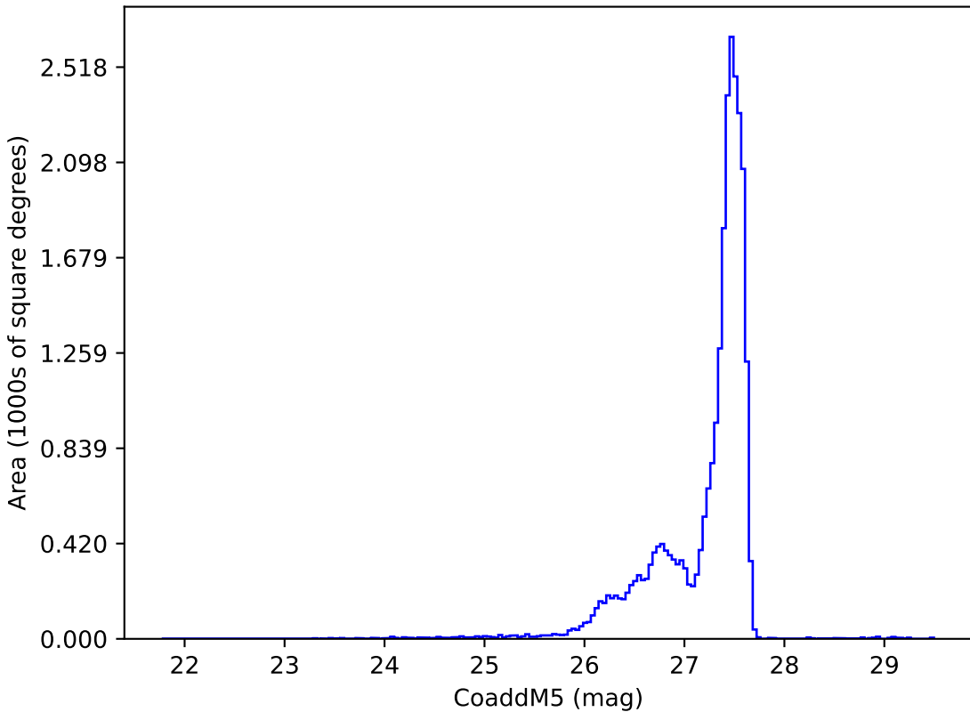
too_elab_r16_d2_ugrizy_v3.4_10yrs : CoaddM5
