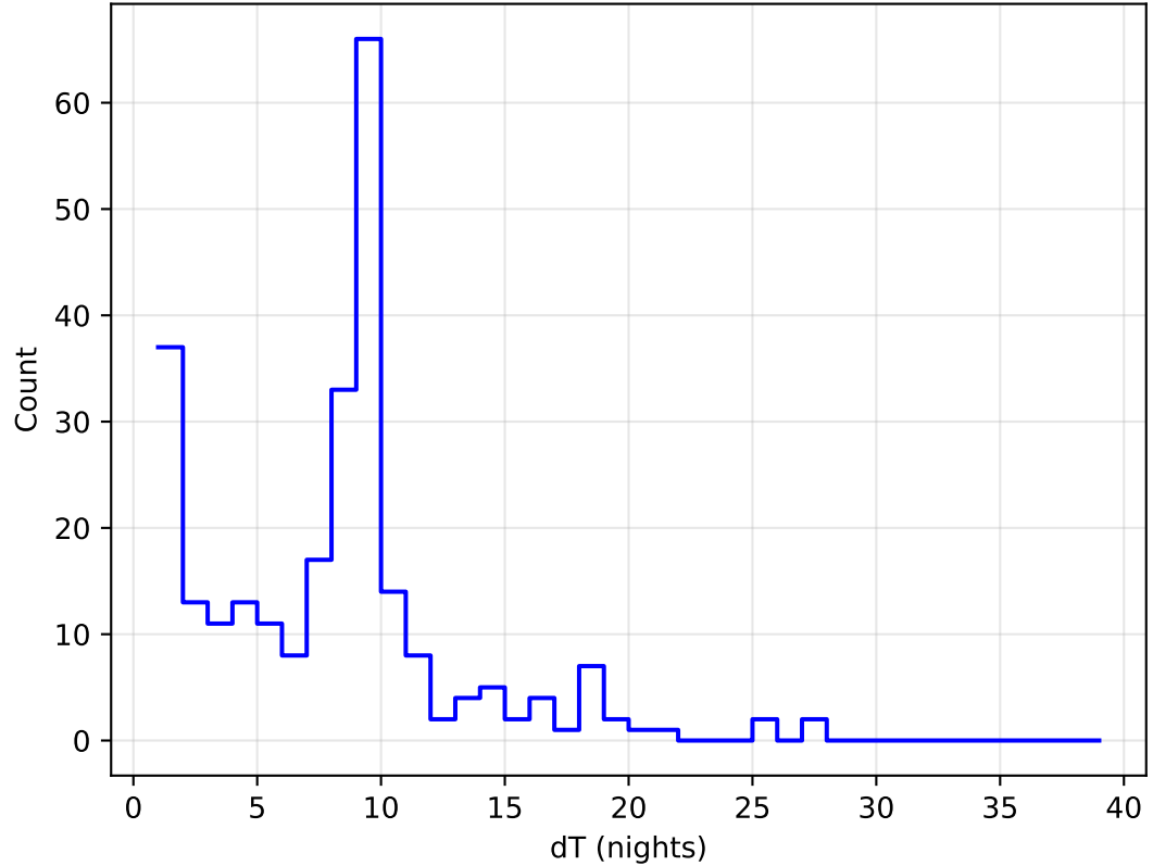
too_elab_r16_d2_ugrizy_v3.4_10yrs all bands: DD:ELAISS1 Delta Nights Histogram
