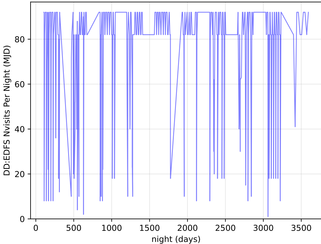
too_elab_r16_d2_ugrizy_v3.4_10yrs all bands: DD:EDFS Nvisits Per Night
