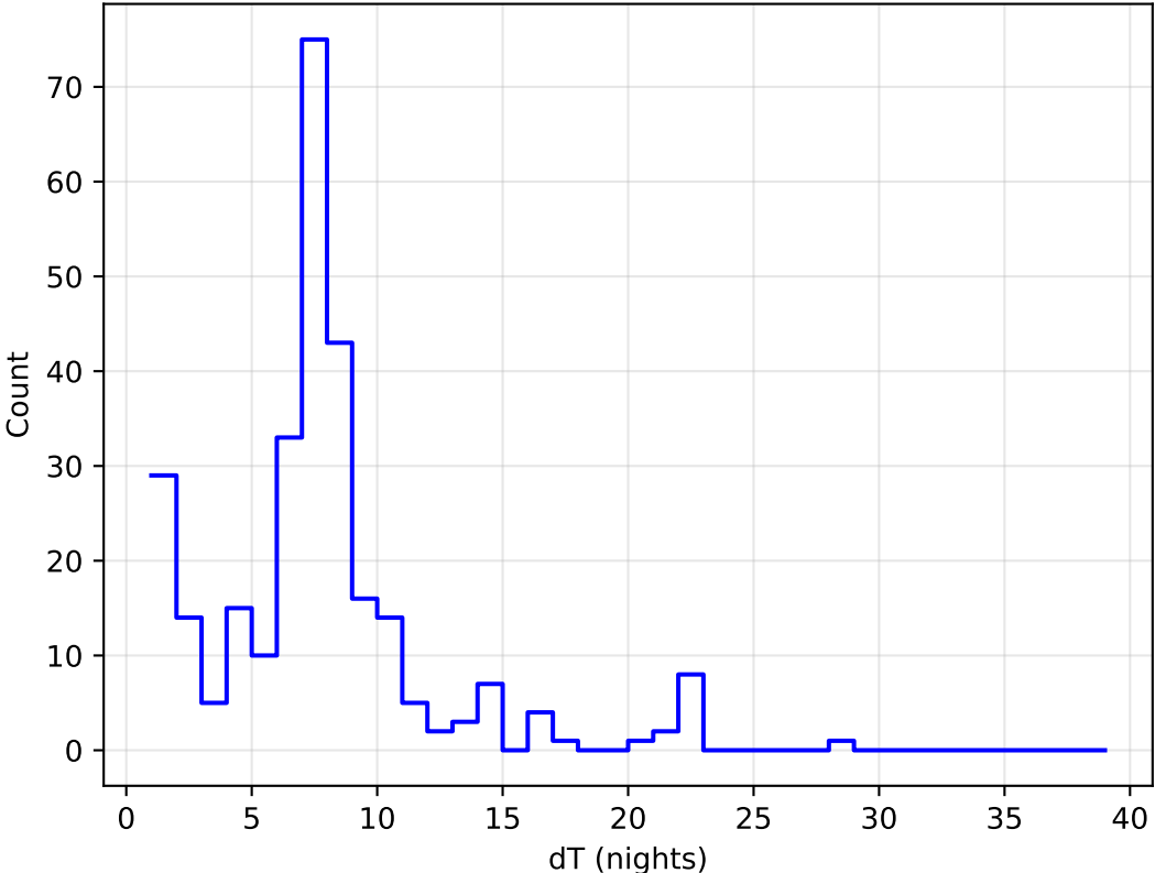
too_elab_r16_d2_ugrizy_v3.4_10yrs all bands: DD:EDFS Delta Nights Histogram
