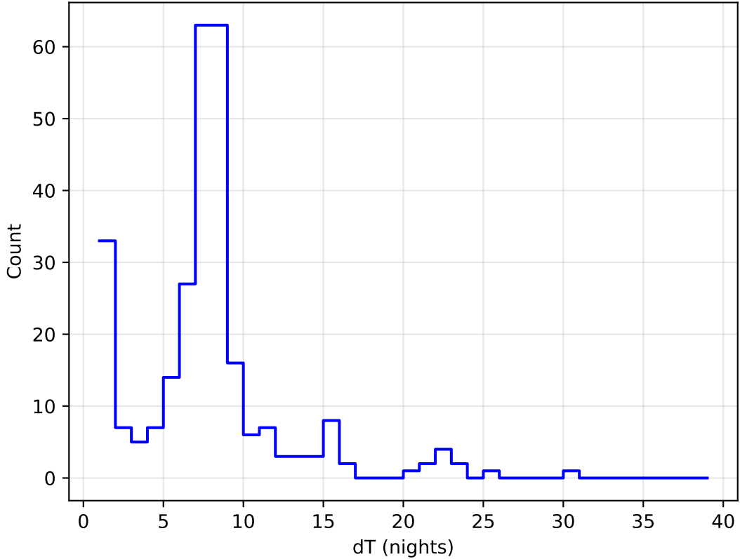
too_elab_r16_d2_ugrizy_v3.4_10yrs all bands: DD:ECDFS Delta Nights Histogram
