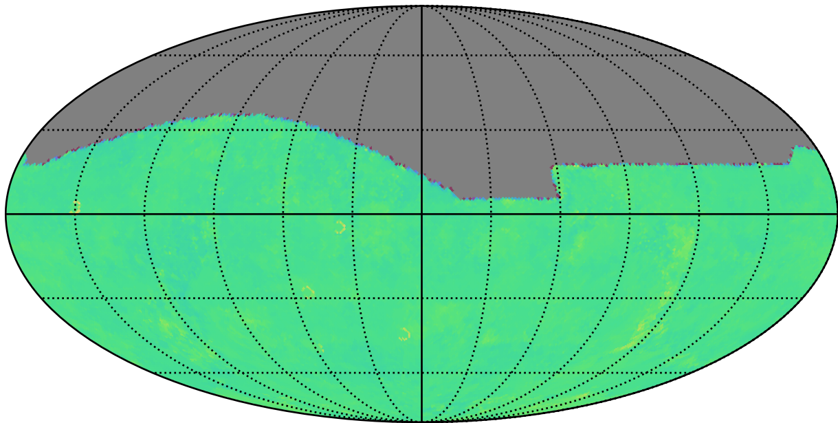
too_elab_r16_d2_gz_v3.4_10yrs g: Kuiper rotTelPos
