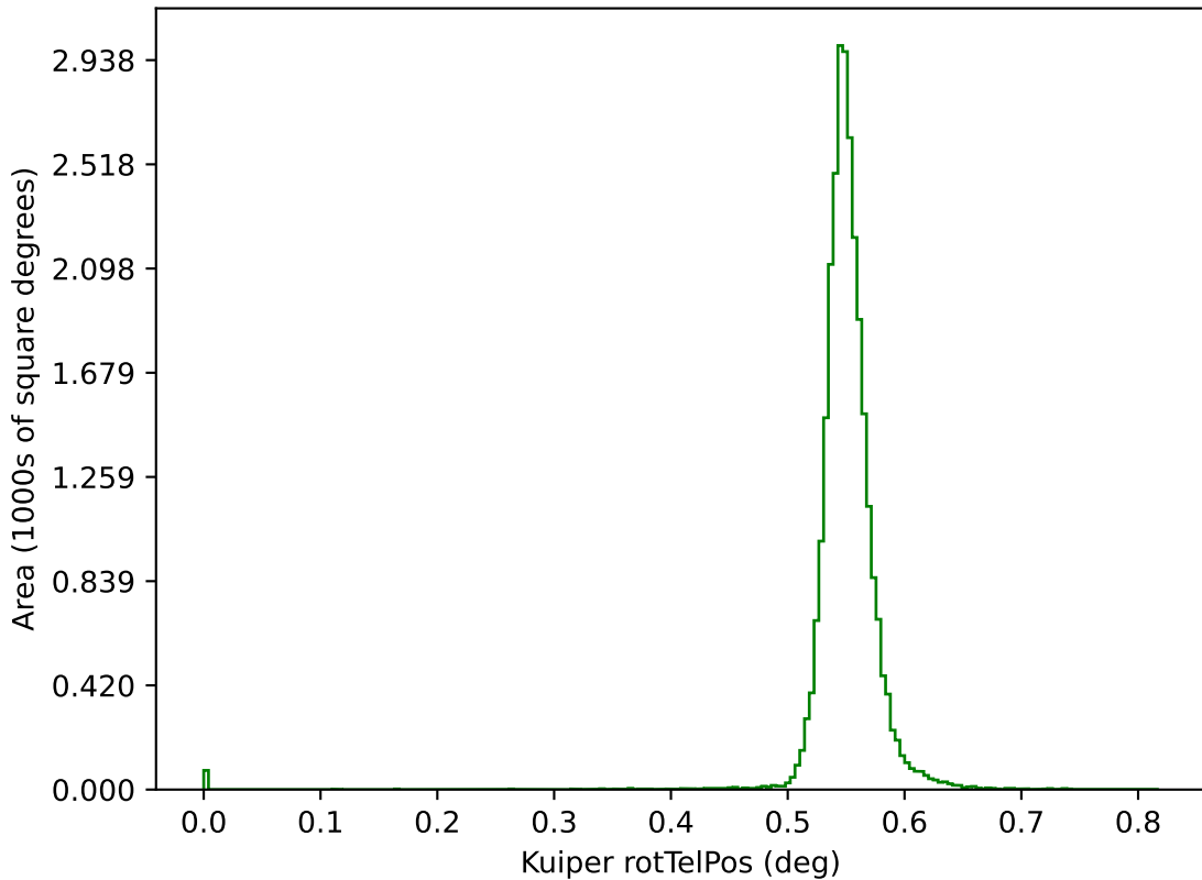
too_elab_r16_d2_gz_v3.4_10yrs g: Kuiper rotTelPos
