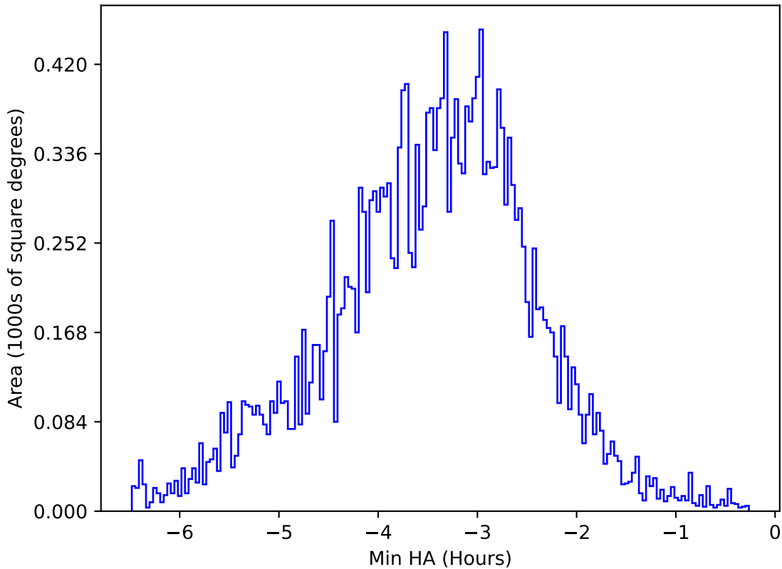
too_elab_r16_d2_gz_v3.4_10yrs All sky y band: Min HA
