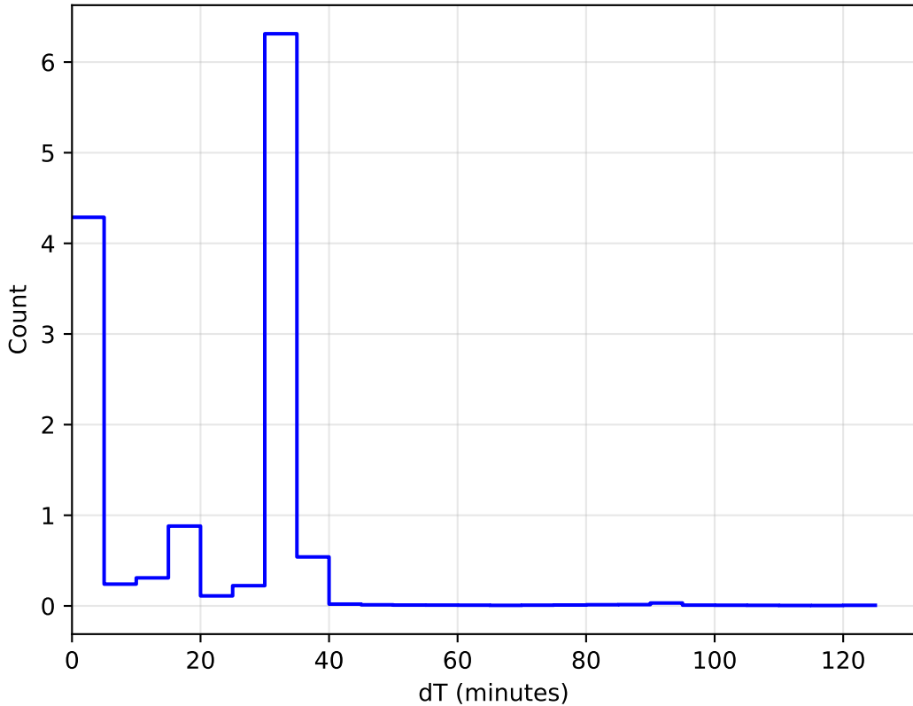
too_elab_r16_d2_gz_v3.4_10yrs All sky: DeltaT Histogram 1e6
