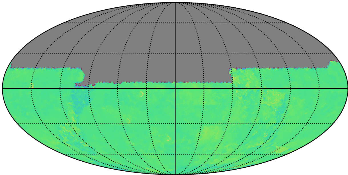
too_elab_r16_d2_griz_v3.4_10yrs u: Kuiper rotTelPos
