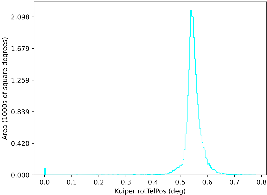
too_elab_r16_d2_griz_v3.4_10yrs u: Kuiper rotTelPos
